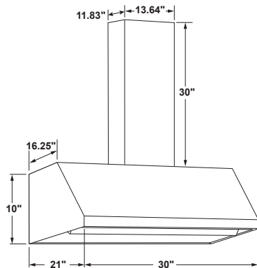
MODEL UVW8304
