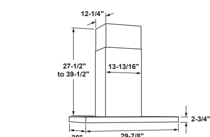
MODEL UVW8301
