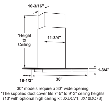
MODEL CVW7301
