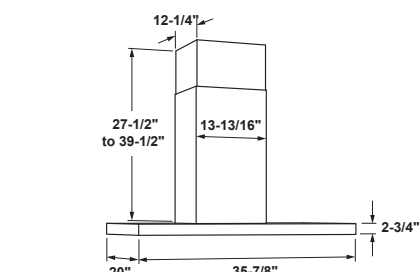
MODEL UVW8361
