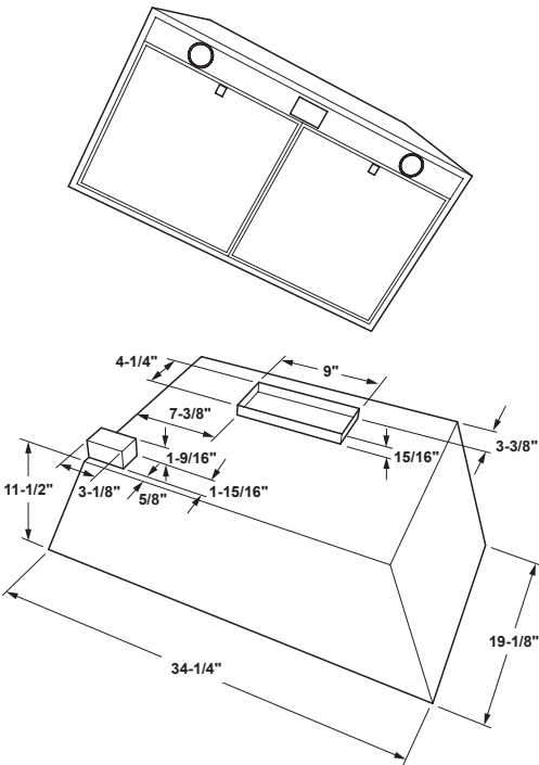
MODEL UVW8304
